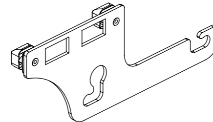
FSS rami prowadz ce lewe 7114401000
