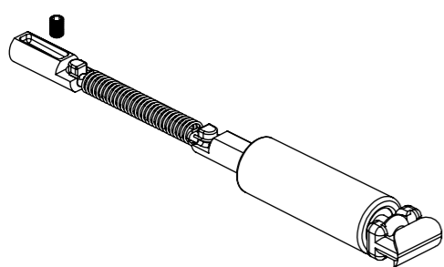
FSS suwak spr ynowy 7110001000
